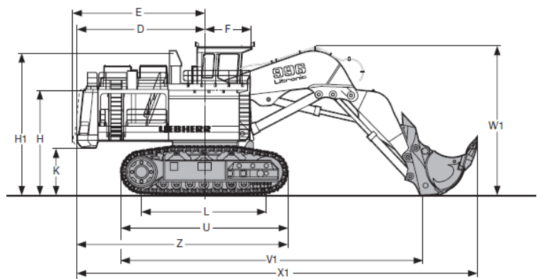
شکل ۱- بیل مکانیکی
