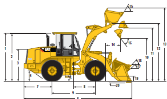
شکل ۲- لودر
